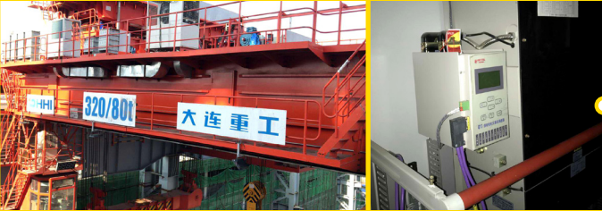
津西钢铁 5 台 320T 铸造吊 主钩电机 400KW×2 QY3-1000S-A-FL 690V 一拖二驱动 具备再启动防溜钩装置
