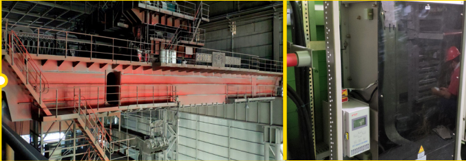
中冶东方重工1台360T铸造吊 主钩电机560KW×2 原ABB调压改造为QY3-2000S-A 690V 一拖二驱动
